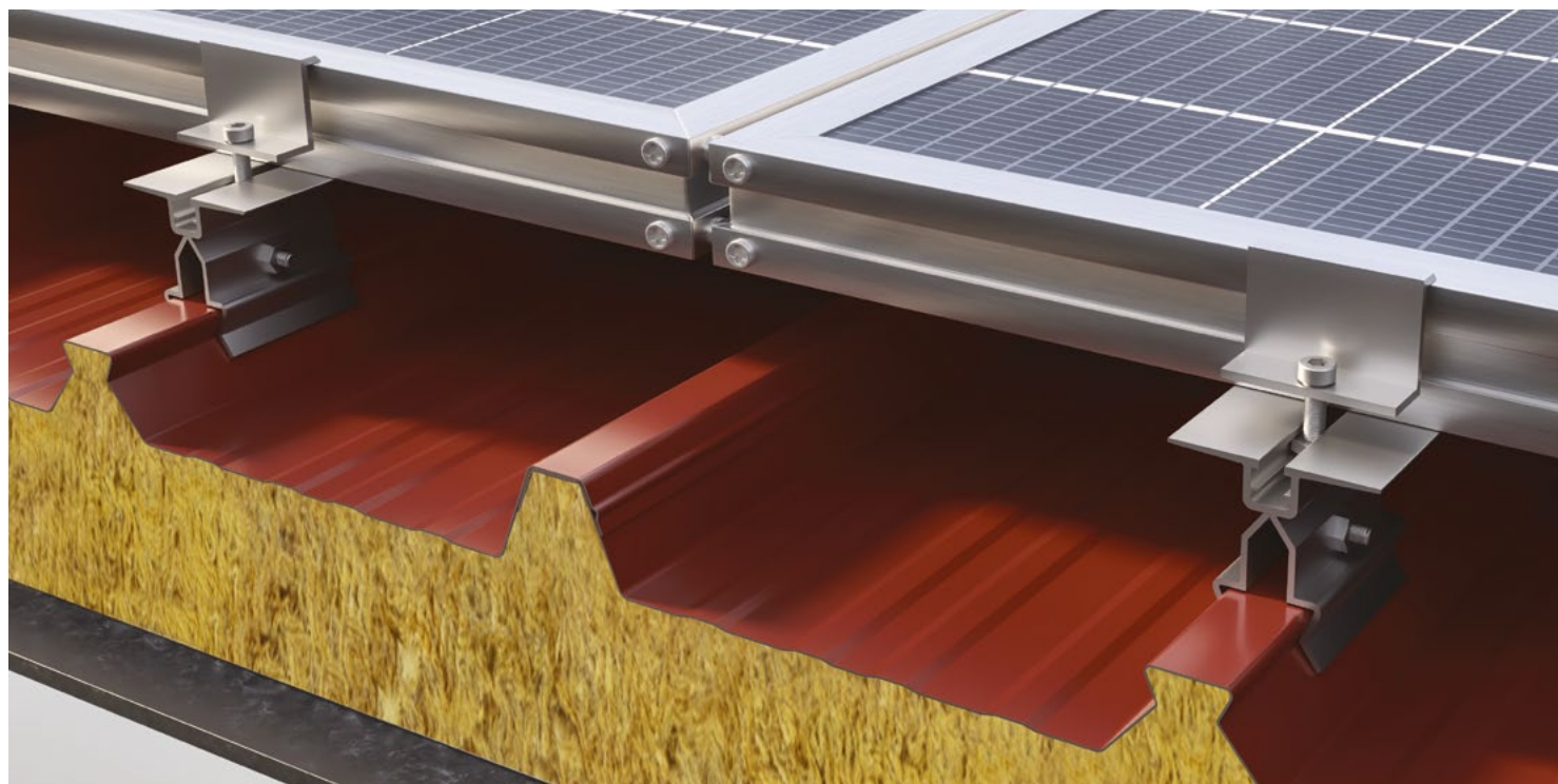
Étrier en aluminium d'accrochage avec fixation OMEGA pour les modules FV avec cadre
