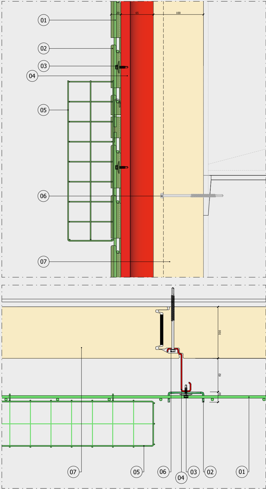
Sezione verticale Vertical section
