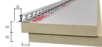
Paneelhoogte 100 mm
