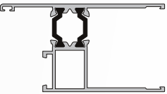
Voorbeeld van een kozijnprofiel met koudebrugonderbreking door een kunststof element
