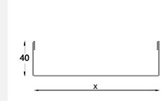
U-vormige gegalaniseerde stalen basis voor panelen van 40 tot 200 mm dik. Andere afmetingen op aanvraag
