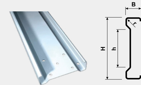
C-profiel
