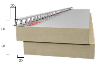
Paneelhoogte 160 mm
