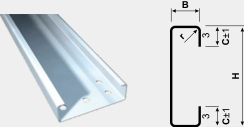
C-profiel
