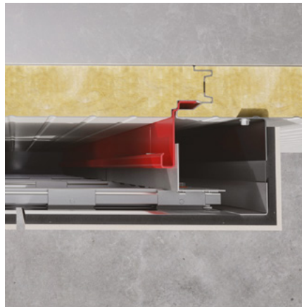
Horizontale doorsnede
