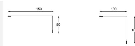
Buitenhoek 150x50mm - 100x100mm. Andere afmetingen op aanvraag
