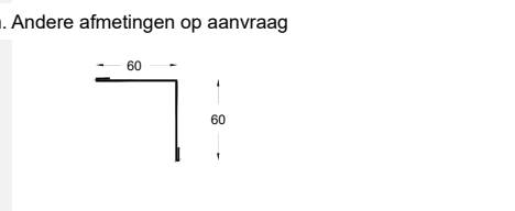
Cornière interieur 60*60mm. Autre dimension sur demande
