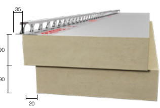
Paneelhoogte 180 mm
