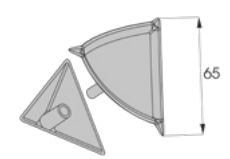
Hoekschaal - mannelijke en vrouwelijke 3-weg pvc-verbindingen
