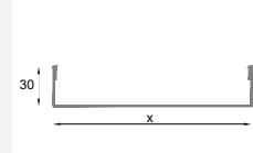
U-vormige stalen bekleding voor panelen van 40 tot 200 mm dik. Andere afmetingen op aanvraag
