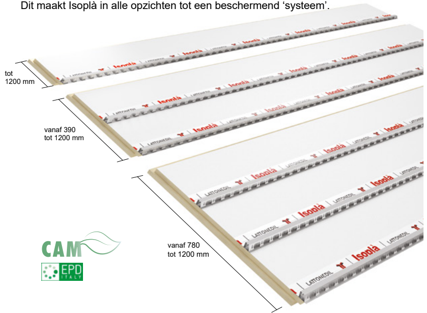
Paneelhoogte 160 mm
