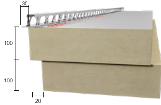
Paneelhoogte 200 mm
