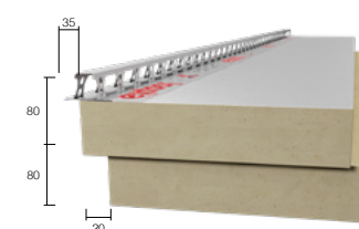
Hauteur panneau 160 mm
