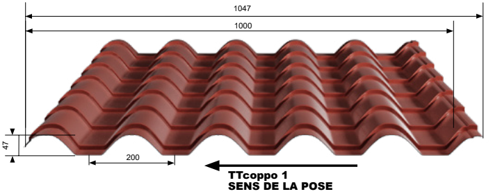
TTcoppo 1 SENS DE LA POSE
