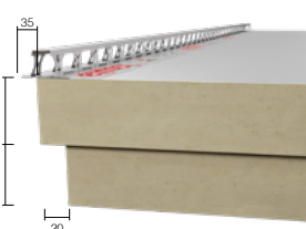
Hauteur panneau 180 mm
