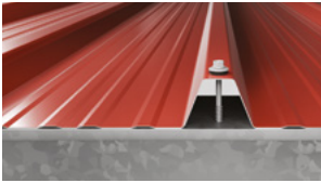
Fixation sur méta
