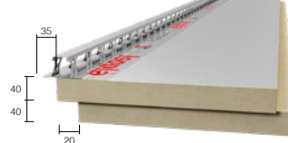
Hauteur panneau 80 mm
