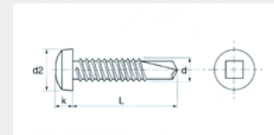
Vis autoperceuses zinguées 4.2*16
