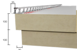
Hauteur panneau 200 mm
