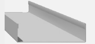
U d'habillage en acier pour panneaux ép. du 40 a 200 mm. Autre dimension sur demande
