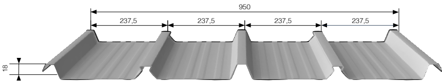
Fixation sur bois
