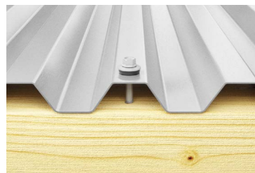
Fissaggio su legno Fastening on wood
